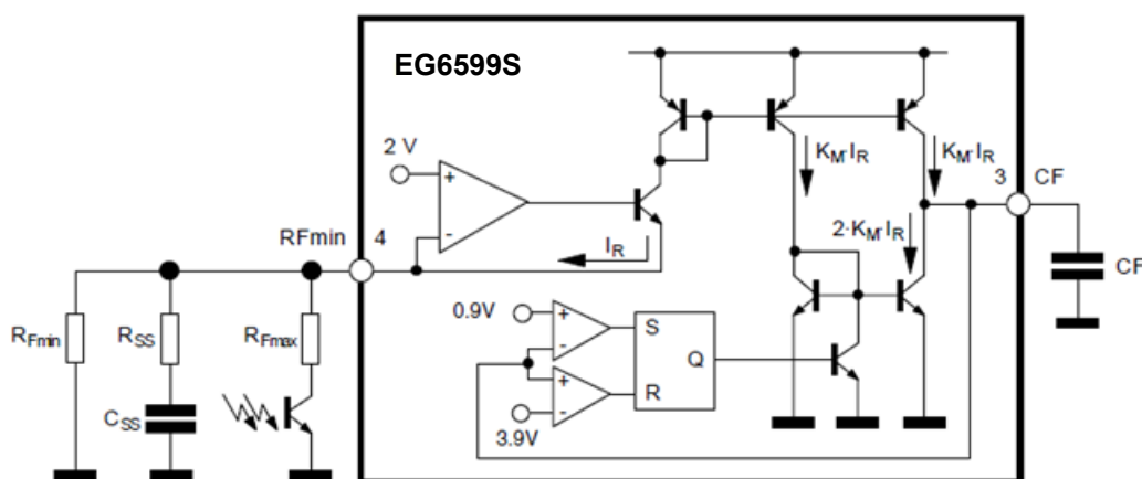
图8-2. 振荡器框图
