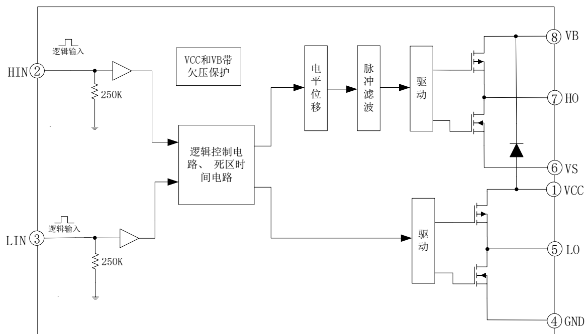
图 5-1. EG2101D 内部电路图
