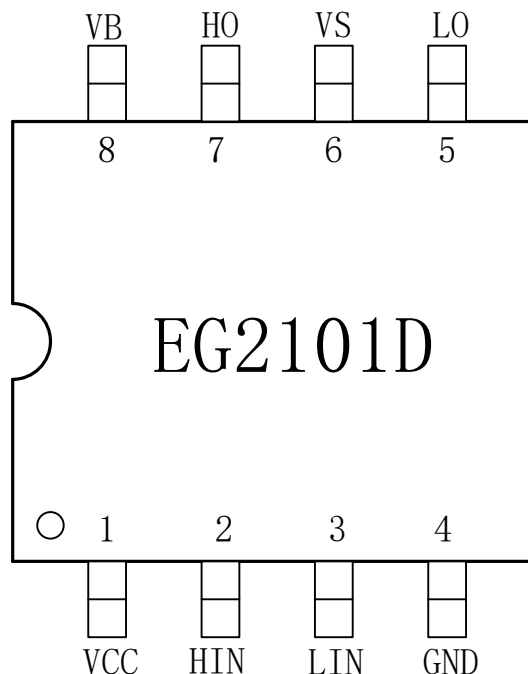
图 4-1. EG2101D 管脚定义
