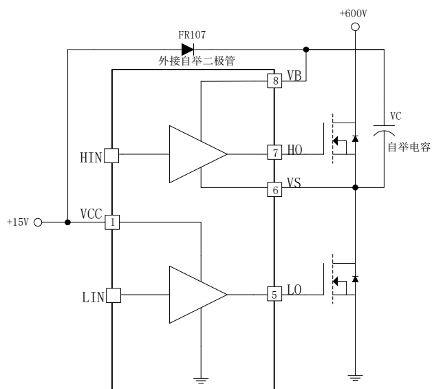
图 8-3. EG2101D 自举电路结构
