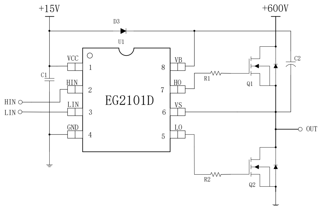
图 6-1. EG2101D 典型应用电路图
