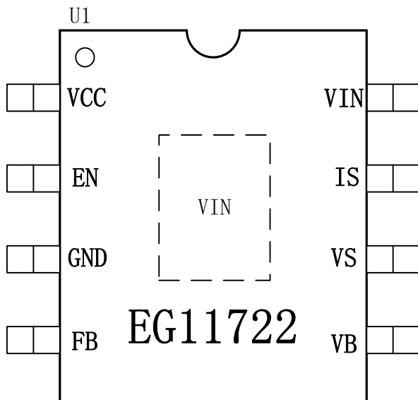
图 4-1. EG11722 管脚定义
