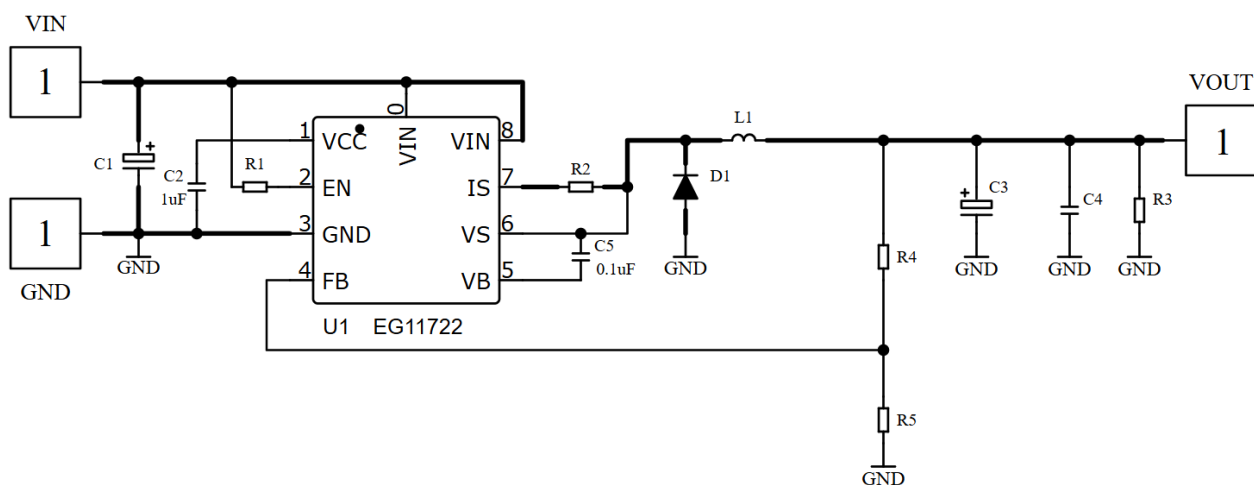
图 6-2. EG11722 5V 或者 3.3V 输出典型应用图，C2、C5 用 25V 耐压足够
