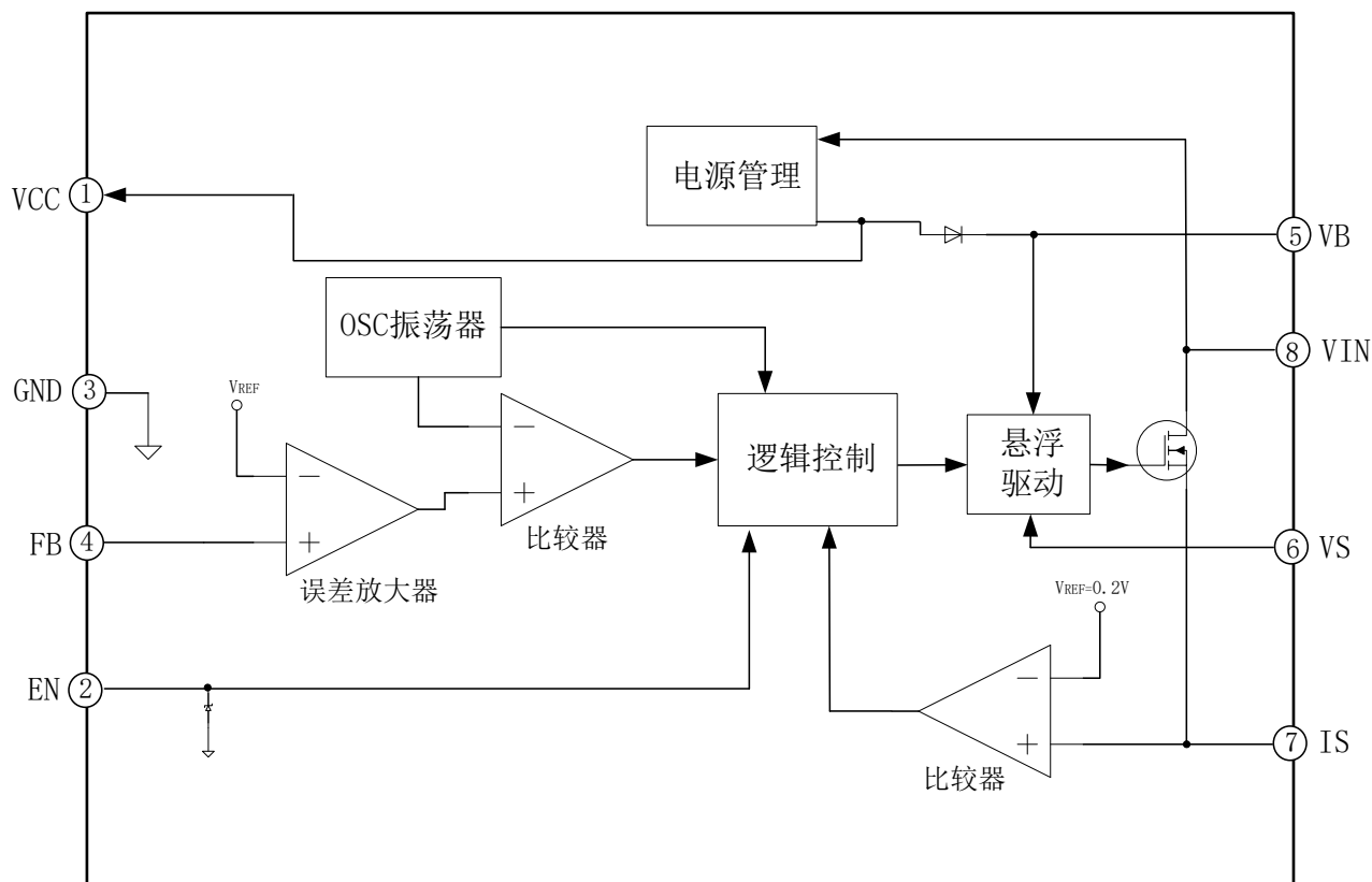
图 5-1. EG11722 内部电路图
