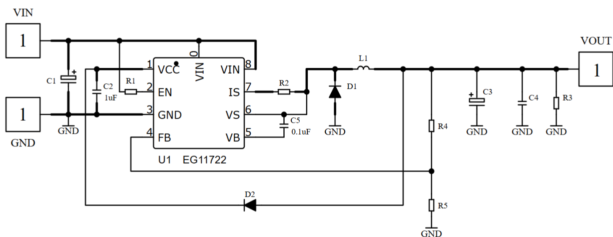
图 6-1. EG11722 12-15V 输出典型应用图，C2、C5 用 25V 耐压足够
