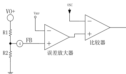
图 8.5 EG11722 输出电压调整电路
