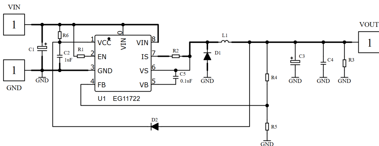
图 6-2. EG11722 宽输入范围典型应用图，C2、C5 用 25V 耐压足够
