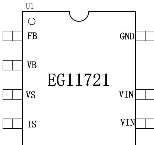
图 4-1. EG11721 管脚定义
