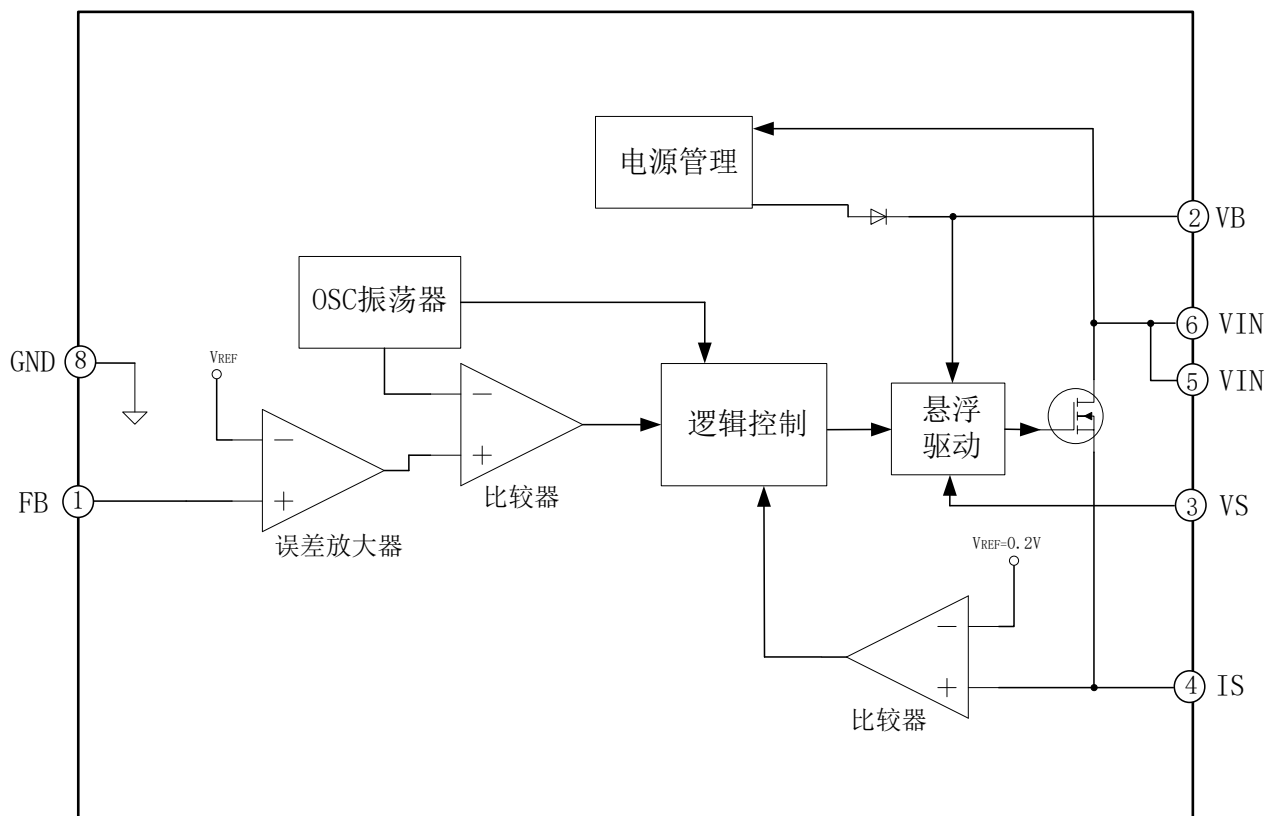
图 5-1. EG11721 内部电路图
