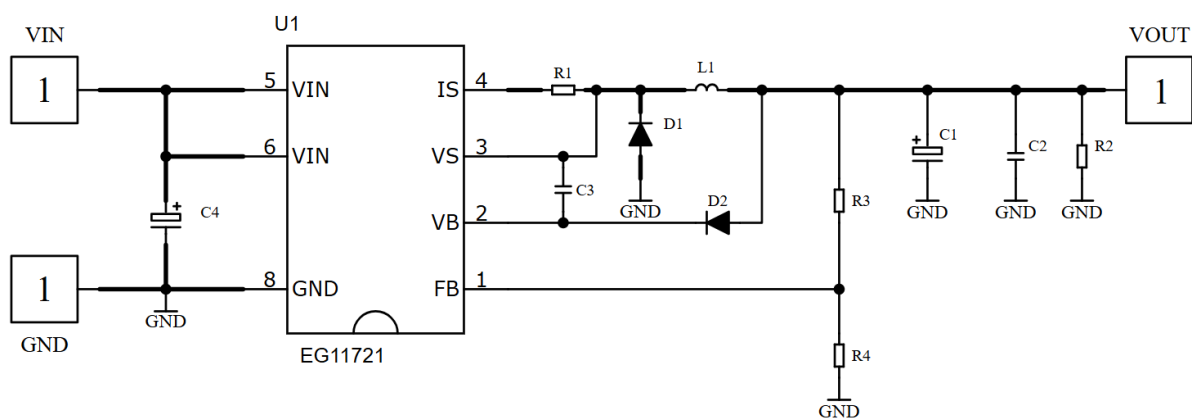
图 6-1. EG11721 12-15V 输出典型应用图，C3 用 25V 耐压足够
