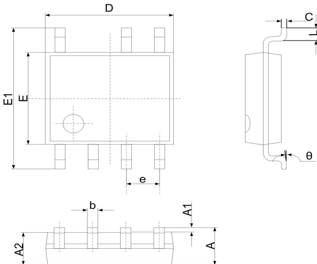
SOP7
