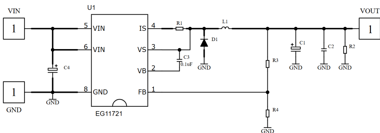
图 6-2. EG11721 5V 输出典型应用图，C3 用 25V 耐压足够
