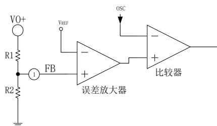
图 8.5 EG11721 输出电压调整电路
