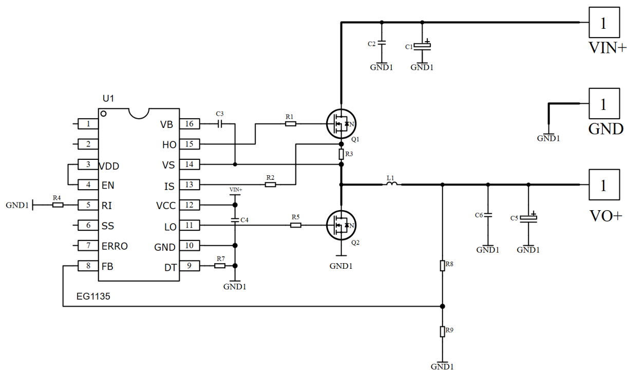
图 6-3. 12V 输入 EG1135 MOS 外置电阻取样典型应用图
