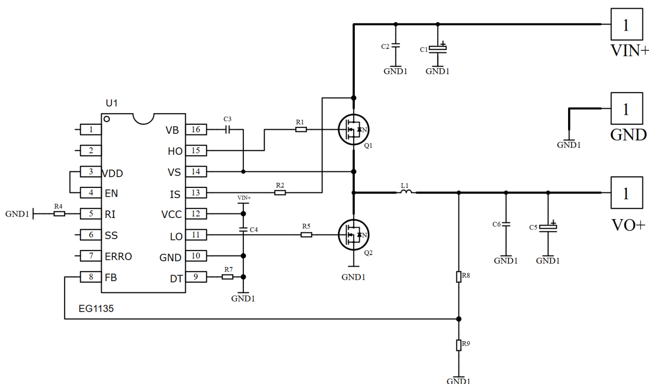
图 6-1. 12V 输入 EG1135 MOS 内置电阻取样典型应用图
