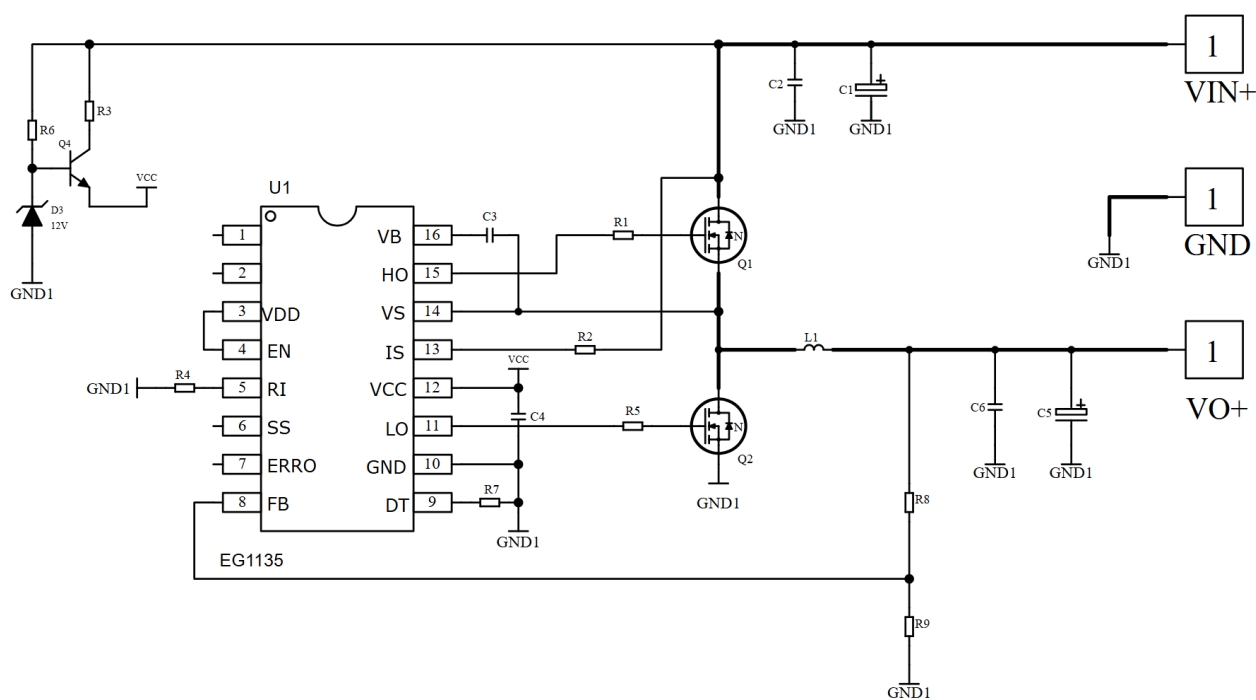
图 6-2. 宽电压输入 EG1135 MOS 内置电阻取样典型应用图
