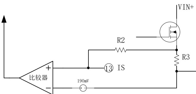
图 8.2 EG1135 峰值限流电路
