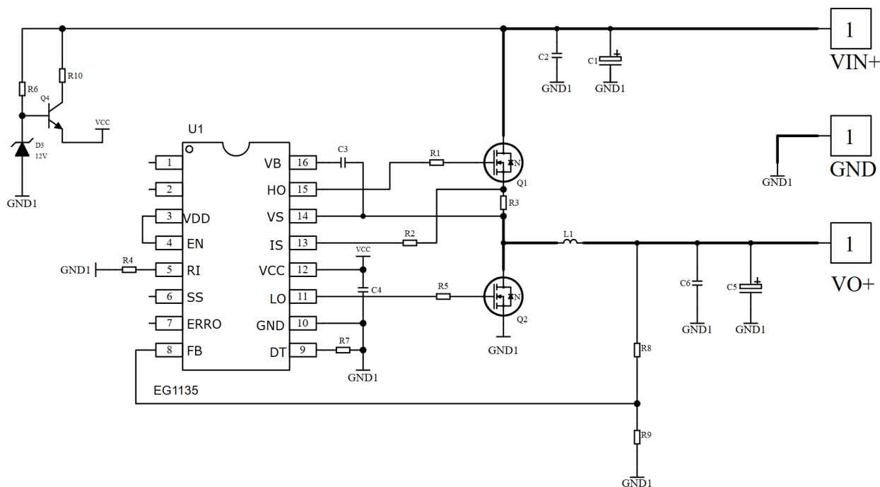
图 6-4. 宽电压输入 EG1135 MOS 外置电阻取样典型应用图
