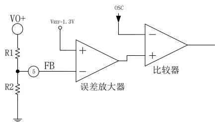
图 8.1 EG1135 输出电压调整电路
