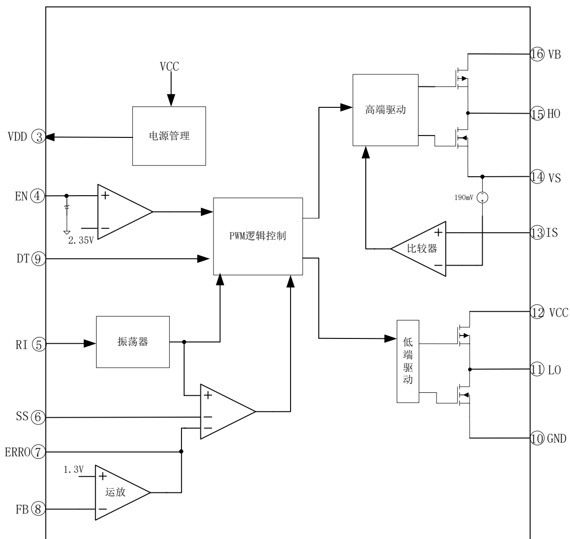
图 5-1. EG1135 内部电路图
