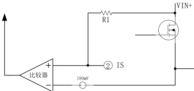
图 8.3 EG11732 功率管内阻峰值限流电路
