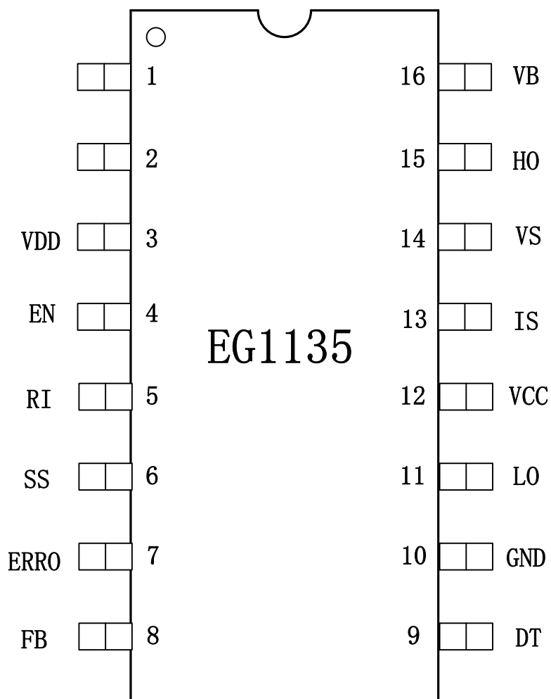
图 4-1. EG1135 管脚定义
